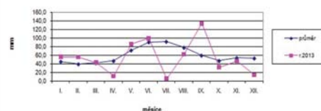
SRÁŽKOVÉ ÚHRNY 1968-2013
