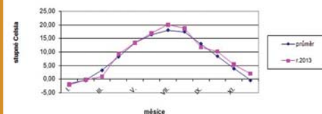
TEPLOTNÍ PRŮMĚRY 1968-2013
