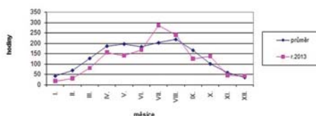
PRŮMĚRNÁ DÉLKA SLUNEČNÍHO SVITU 2008 AŽ 2013 A ROKU 2013
