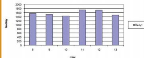
SLUNEČNÍ SVIT 2008 AŽ 2013
