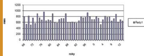
SRÁŽKOVÉ ÚHRNY 1968-2013
