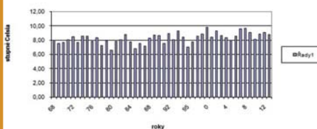
TEPLOTNÍ PRŮMĚRY 1968-2013
