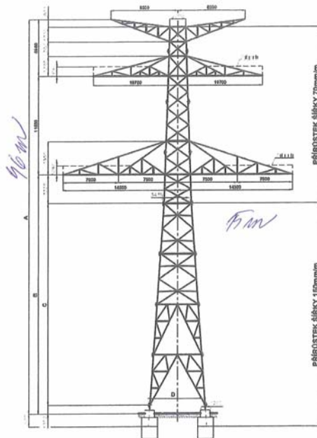
Obrázek č.1 - Stožár typu DUNAJ
